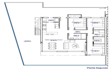
Planta Segunda E: 1/150
