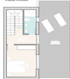
Planta Primera
